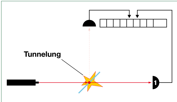
Tunnelt das Photon den Spiegel, so wird es von dem dahinter liegenden Detektor erkannt und die Auswertungseinheit erhält eine 1.
