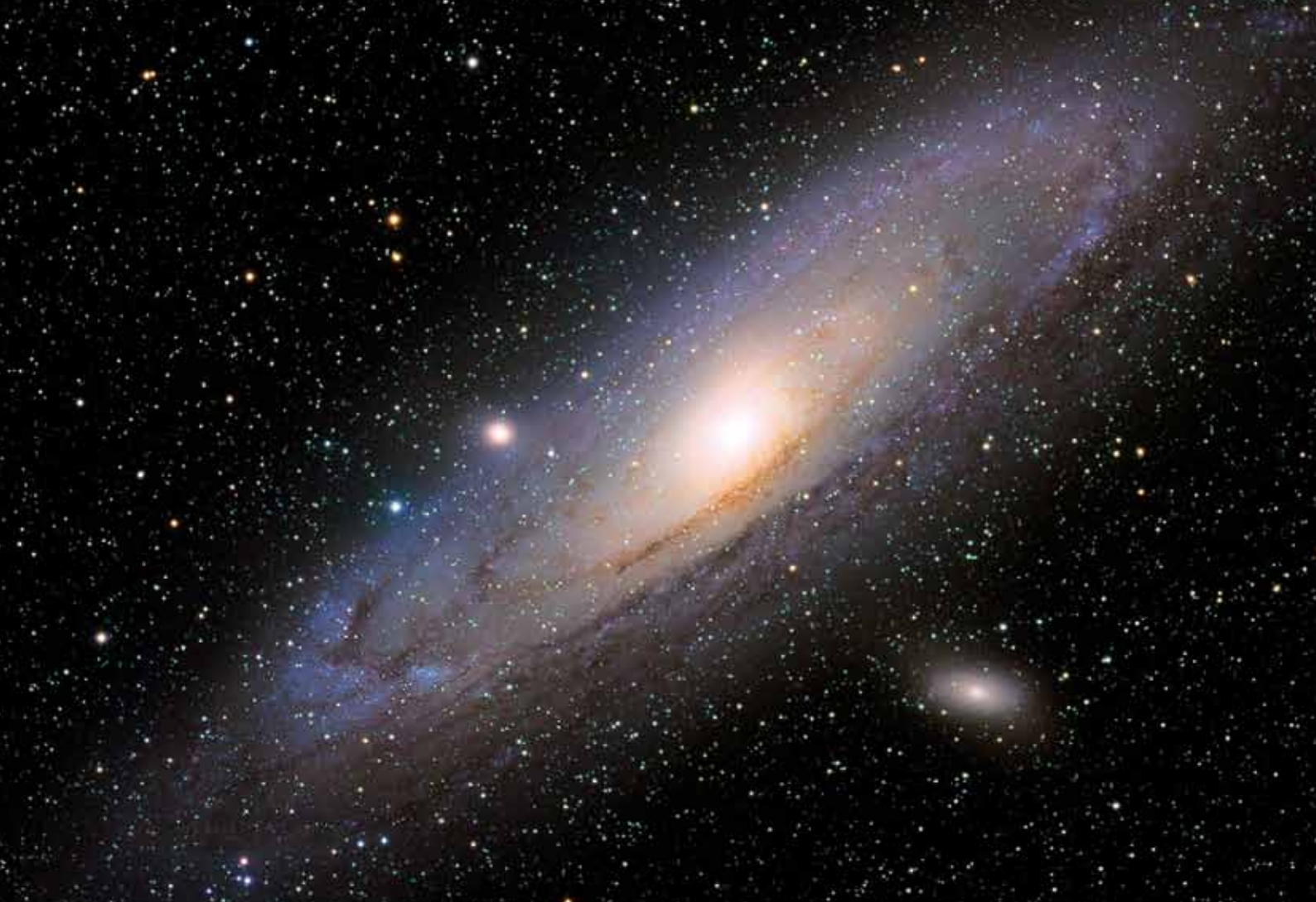
Andromeda Galaxie M31
