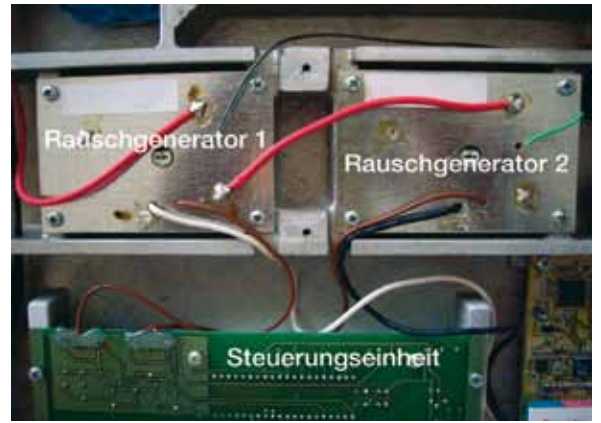
Rauschquellen, die ein verwertbares Signal liefern sollen, müssen sorgfältig gegen elektromagnetische Strahlung abgeschirmt werden.
