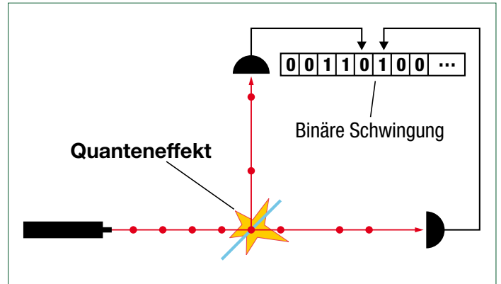
Die auf diese Weise erzeugte hochfrequente binäre Zahlenfolge ist absolut nicht-deterministisch und daher ideal zur Informationsfeld-Kommunikation geeignet.
